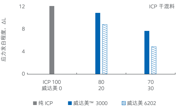
威达美减轻应力发白
