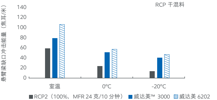
抗冲击强度 – 在 RCP 中加入 10% 的威达美
