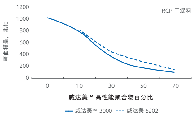
弯曲模量
