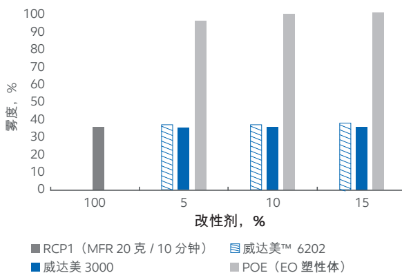
光学性能 – 改性剂聚合物与 RCP 的共混物制成的 1 毫米厚圆盘
