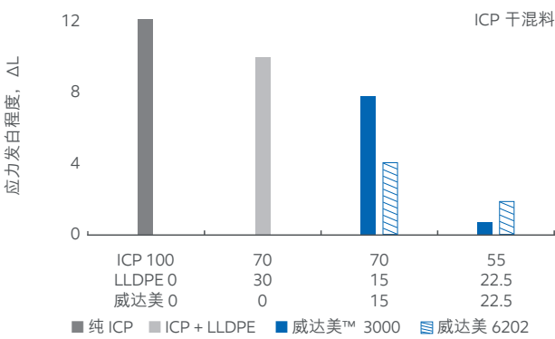
威达美和 LLDPE 减轻应力发白
