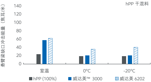
抗冲击强度 – 在 hPP 中加入 10% 的威达美
