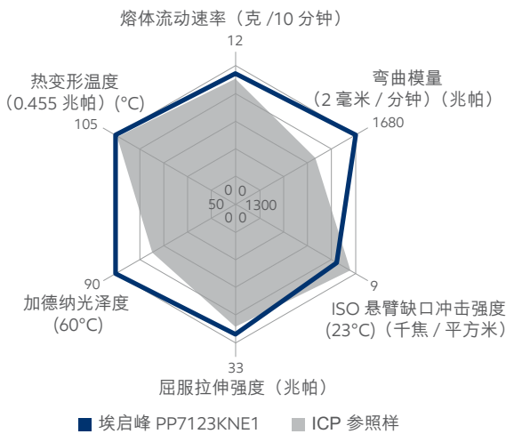
图 1 : 埃启峰 PP7123KNE1 与参照抗冲共聚聚丙烯 (ICP) 的主要性能数据对比。主要凸显提升的美观性。
