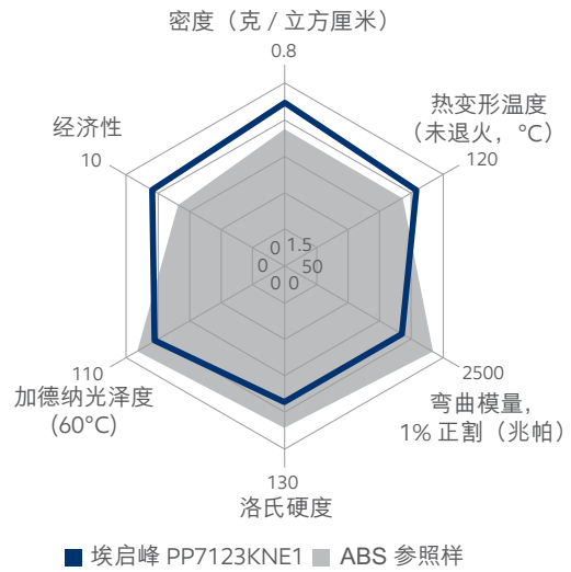
图 2 : 埃启峰 PP7123KNE1 与参照 ABS 的主要性能数据对比。主要凸显成本节约。
